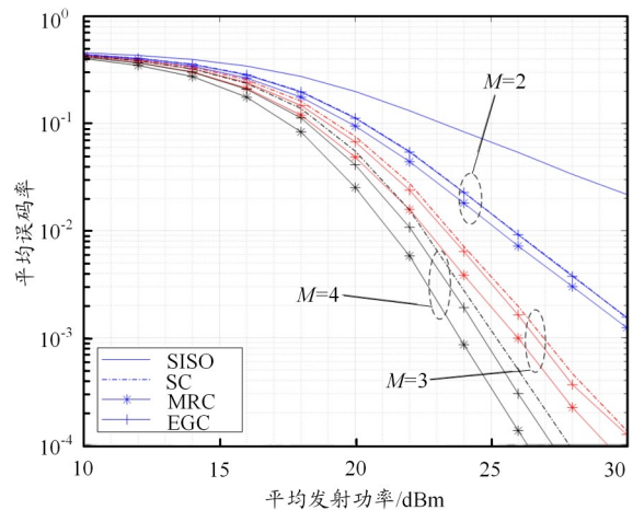
图9 弱湍流环境下,SC/MRC/EGC分集
